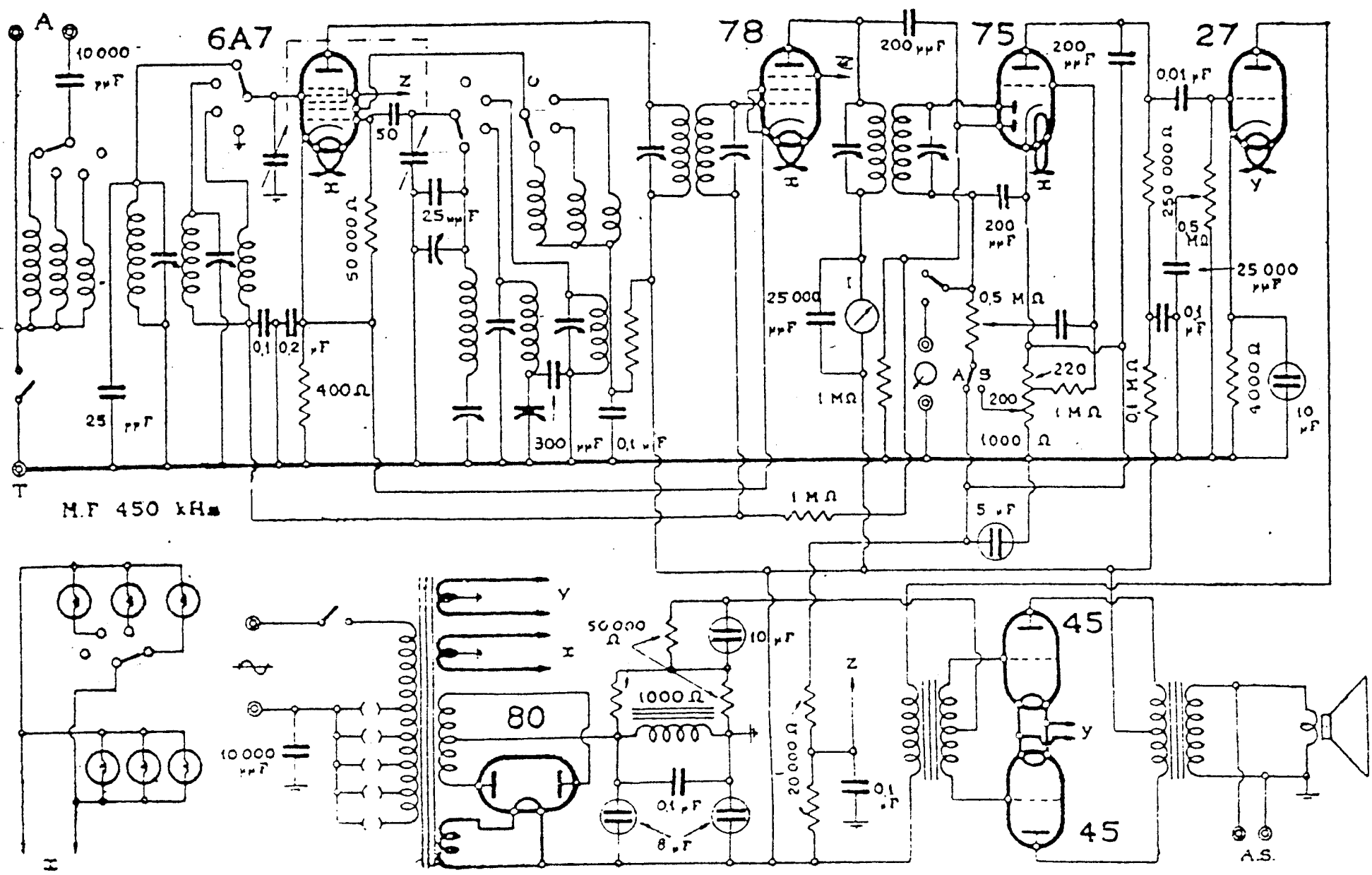
UNDA RADIO - MODD. « TRI UNDA 700 » « 707 »
